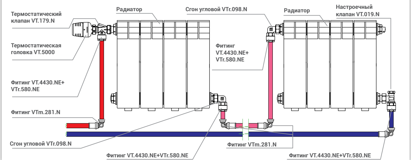
Рис. 24 Последовательное подключение приборов при комбинированной схеме
